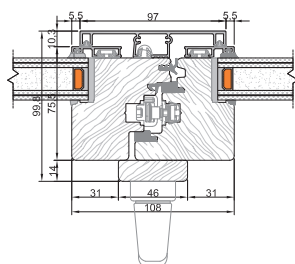
Mittlerer Knoten Innenliegende Abdeckleiste, Eintritt 0
