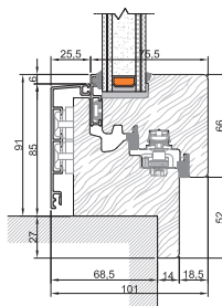
Mittlerer Knoten Innenliegende Abdeckleiste, Eintritt 0
