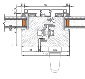
Mittlerer Knoten Standard
