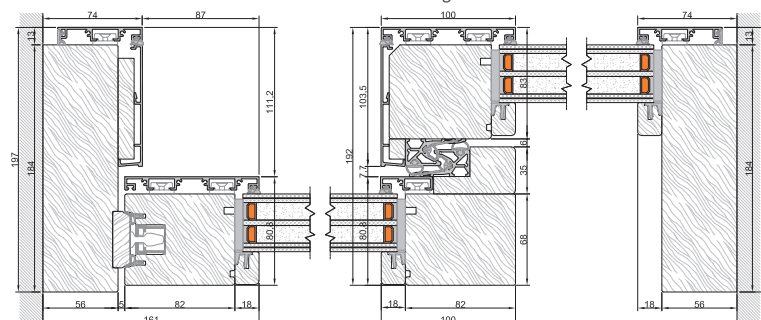
Mittlerer Knoten Panorama-Flügel
