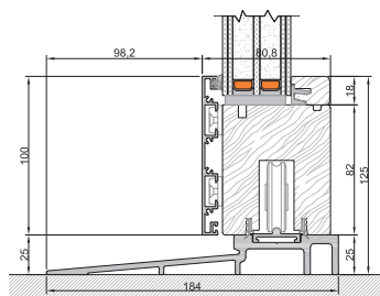
Unterer Knoten Flügel mit Schwelle
