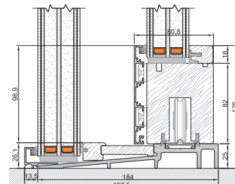
Unterer Knoten Panorama-Flügel
