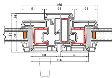
Mittelknoten Eckiger Flügel
