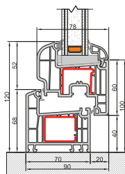
Unterer Knoten Abgerundeter Flügel mit Rahmen L
