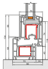
Unterer Knoten Vergrößerter Flügel mit Rahmen L
