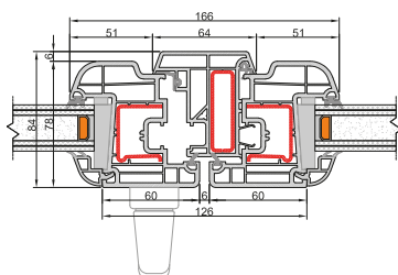
Mittelknoten Abgerundeter Flügel
