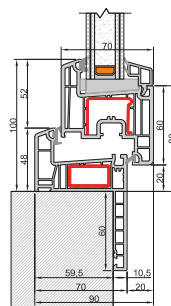
Mittelknoten Eckiger Flügel
