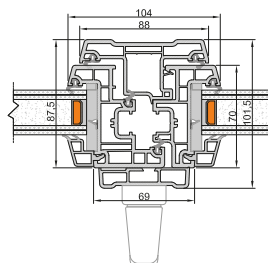
Mittelknoten Sistema P70 EVO DESIGN
