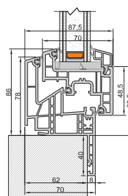
Unterer Knoten Rahmen Z40
