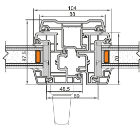
Mittelknoten Sistema P70 EVO
