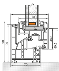
Unterer Knoten Rahmen L
