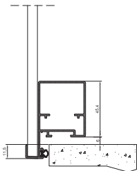
Unterer Knoten Anschlagflügel
