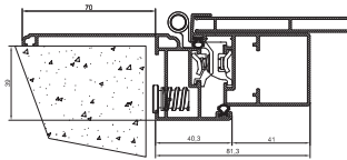
Seitlicher Knoten Rahmen Z70
