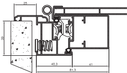
Seitlicher Knoten Rahmen Z25
