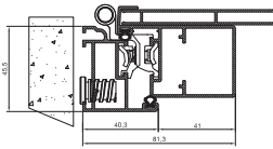
Seitlicher Knoten Rahmen L
