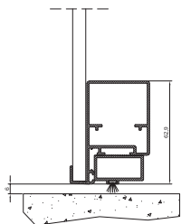
Unterer Knoten Flügel bündig
