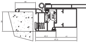
Seitlicher Knoten Rahmen Z40
