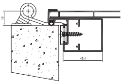
Seitlicher Knoten Anschlagflügel
