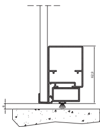
Unterer Knoten Flügel bündig
