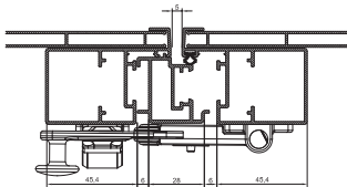
Unterer Knoten Anschlagflügel
