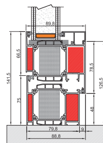
Unterer Knoten Verstärkter Flügel und Rahmen L
