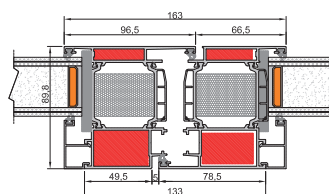
Mittelknoten Verstärkter Flügel
