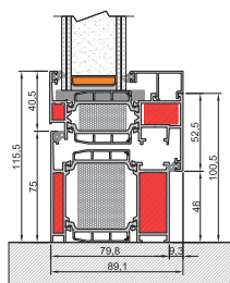
Unterer Knoten Verstärkter Rahmen L
