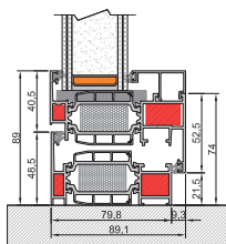
Unterer Knoten Rahmen L
