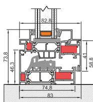
Unterer Knoten Rahmen L
