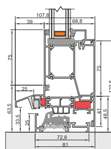
Unterer Knoten Abgesenkte Schwelle
