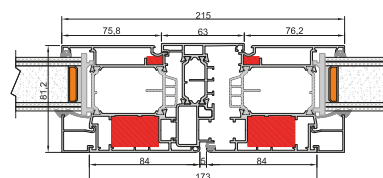
Mittelknoten Verstärkter Flügel
