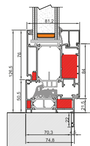
Unterer Knoten Verstärkter Flügel mit Rahmen Z22
