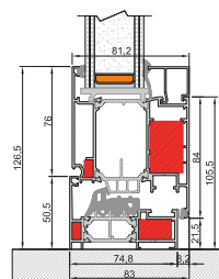
Unterer Knoten Verstärkter Flügel mit Rahmen L
