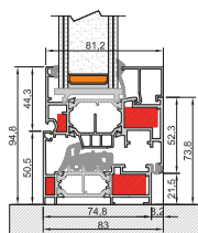
Unterer Knoten Rahmen L
