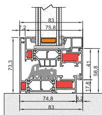
Unterer Knoten Rahmen L
