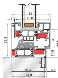
Unterer Knoten Rahmen Z22
